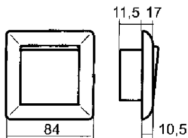
Målskisse
