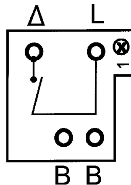
Koblingsskjema
