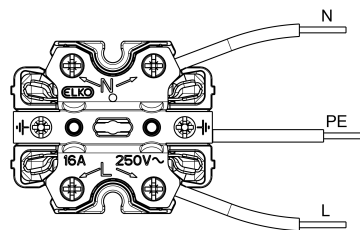
Koblingsskjema
