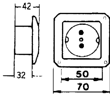
Målskisse
