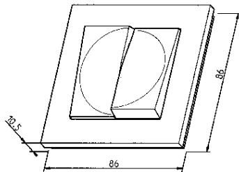
Målskisse
