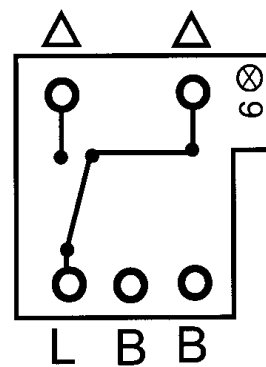
Koblingsskjema
