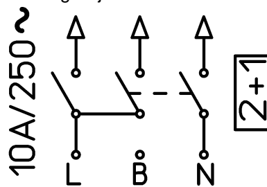
Koblingsskjema
