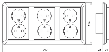
Målskisse
