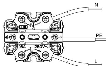
Koblingsskjema
