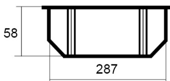
Målskisse
