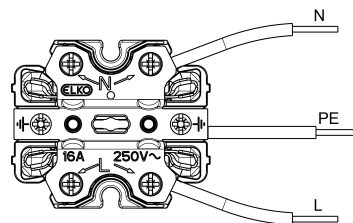
Koblingskjema
