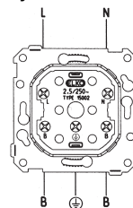
Koblingsskjema
