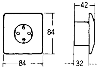
Målskisse
